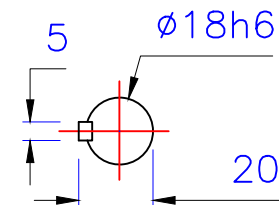
出力轴 Output shaft
